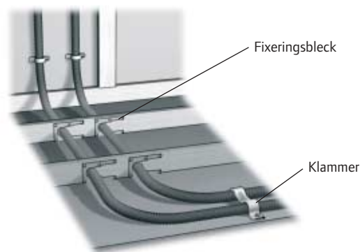
Förslag till placering av rör i regler.
