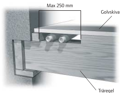
Förslag till placering av rör längs yttrevägg.
