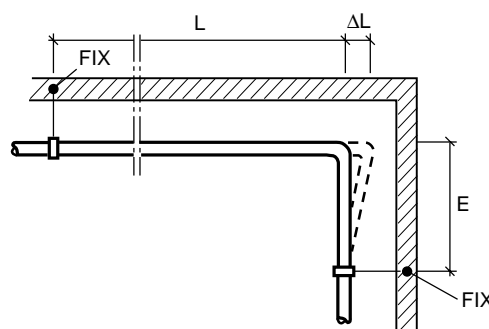
Expansionsanordning vid riktningssändring.
