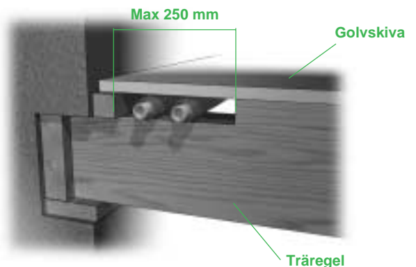
Förslag till placering av rör längs yttervägg.
