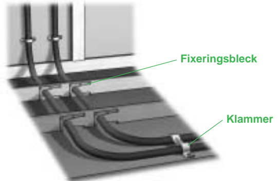
Förslag till placering av rör i regler.
