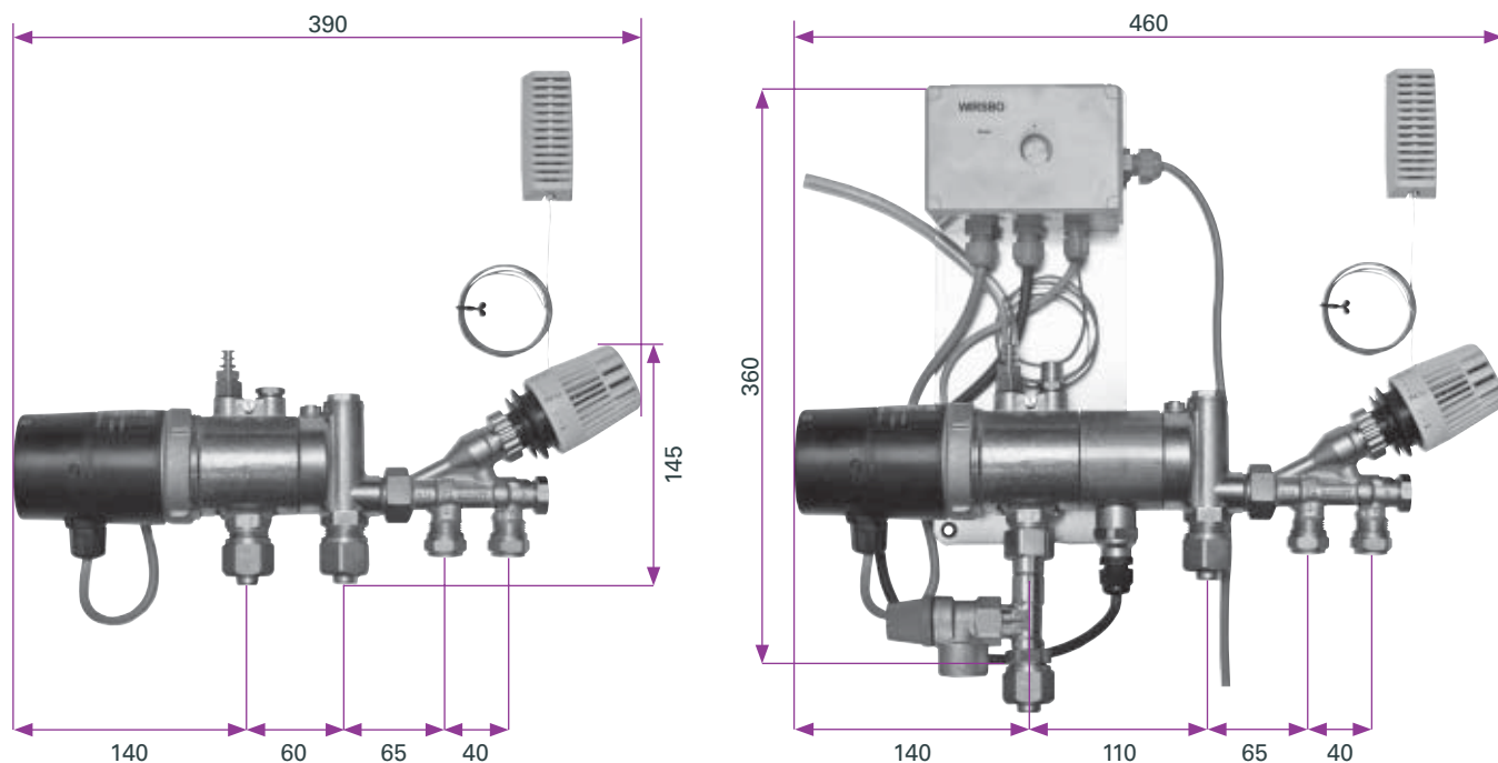
Fig 5 Alla mått angivna i mm. Avstånd från vägg till centrum rör 45 mm. Totalt byggdjup 78 mm för Uponor Push 12, motsvarande byggdjup för Uponor EIPush12 är 105 mm. Anslutning primärkrets \varnothing 15 mm, sekundärkrets PEX 20x2 mm
