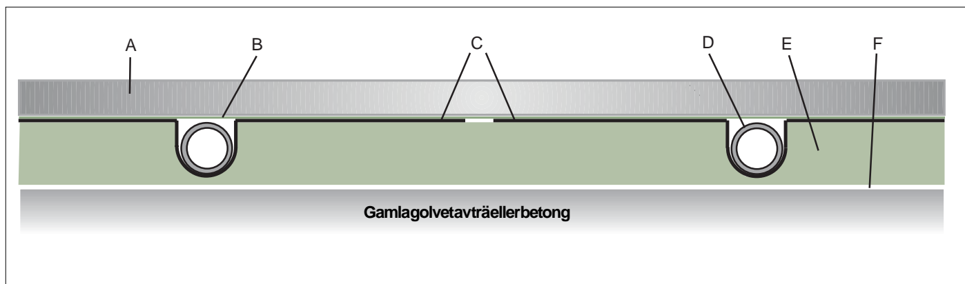
Principiell uppbyggnad av Wirso Golvvärme 12 med golvvärmeskiva.
