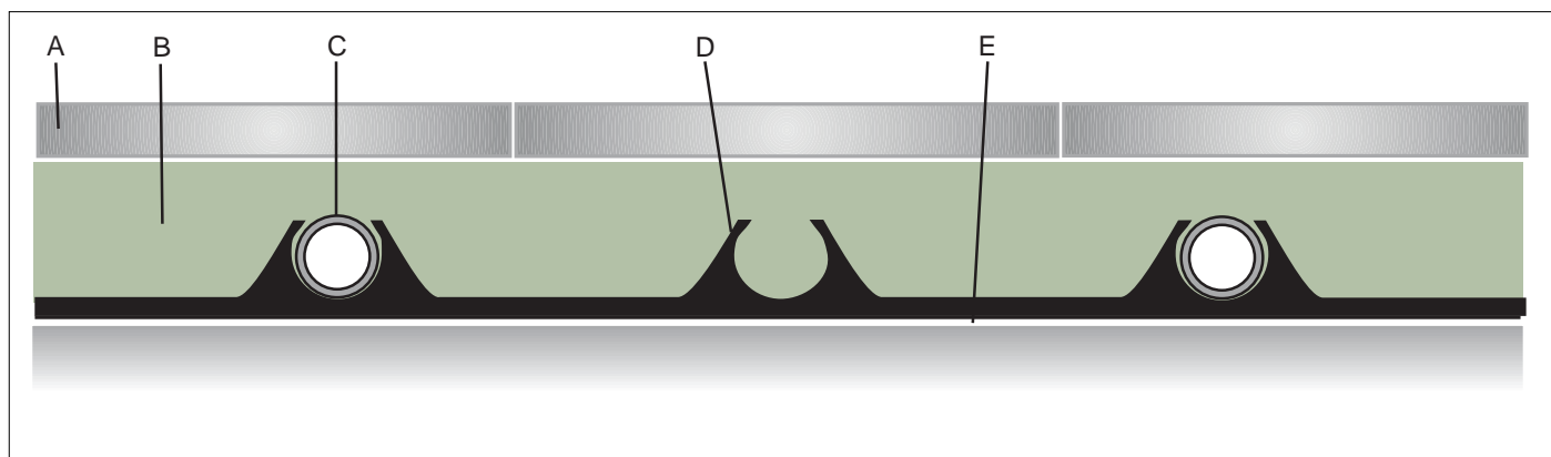
Principiell uppbyggnad av Wirso Golvvärme 12 med rörhållarskena.
