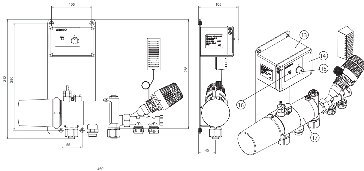
Fig 9 Skiss på Uponor ElPush12 med radiatorventil.
